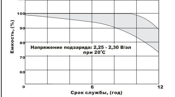
Срок службы в буферном режиме
