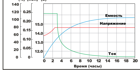
Заряд постоянным напряжением (0.25СA, 20°C)
