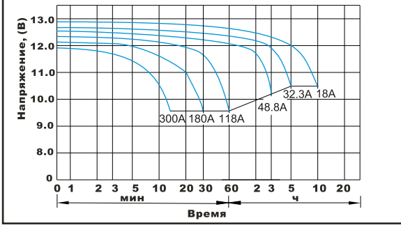
Разрядные характеристики (20°C)
