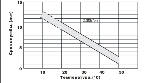
Влияние температуры на срок службы
