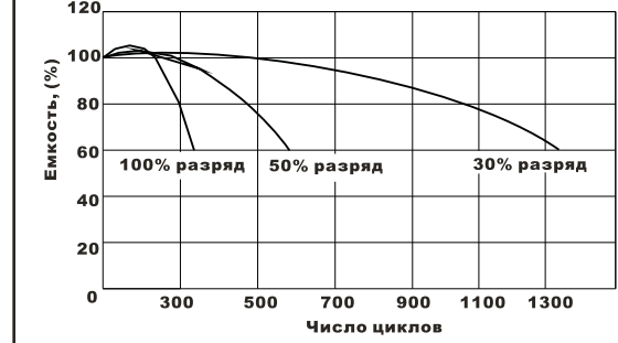
Срок службы в циклическом режиме
