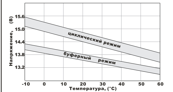
Влияние температуры на напряжение заряда
