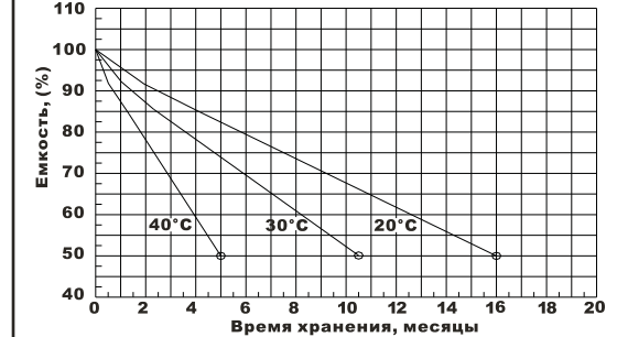
Саморазряд
